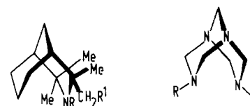
228a R=O R 1 =I 228b R=O R 1 =H 229 R=NO 230 R=NO 2
